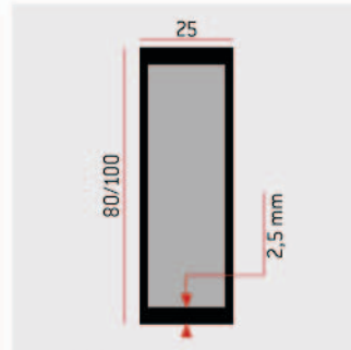
Verstärkte Profile 2,5 mm. Profils à section renforcée 2,5 mm.
