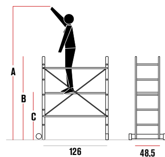
Ruota da 80 mm. per facilitare gli spostamenti. 80 mm wheel facilitates displacement.
