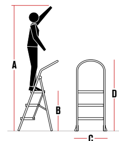
Sicurezza superiore con il sistema di stabilizzazione a croce. Top safety guaranteed by the cross-stabilising system.
